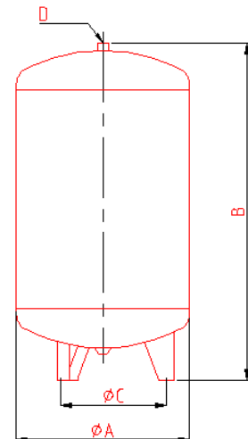
110 - 1000 Litres
